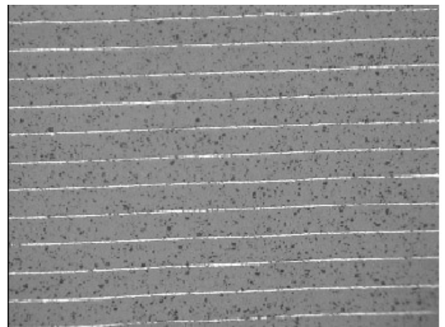
MLCC 断面 SEM 图 MLCC Fracture Surface SEM
